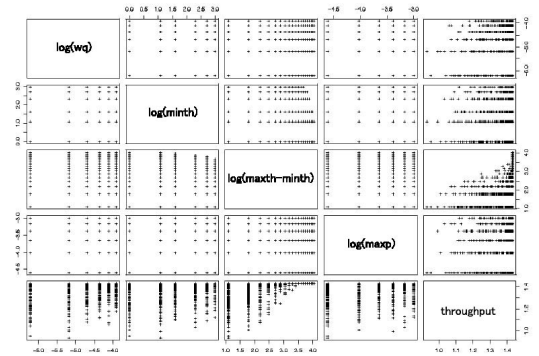
図5 REDのスループットに関する多変量相関図 (変数変換後) Fig. 5 Pair scatter plot of control parameters and throughput (with variable transformation)
