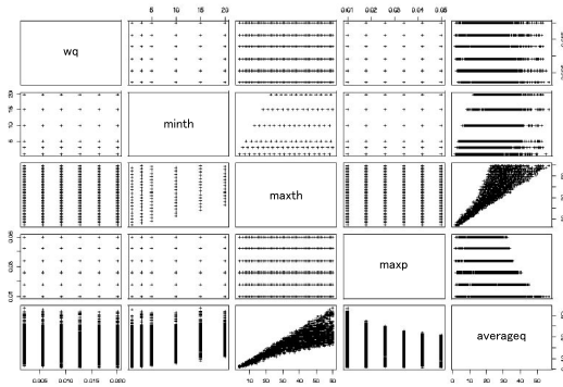
図4 REDの平均キュー長に関する多変量相関図 Fig. 4 Pair scatter plot of control parameters and average queue length
