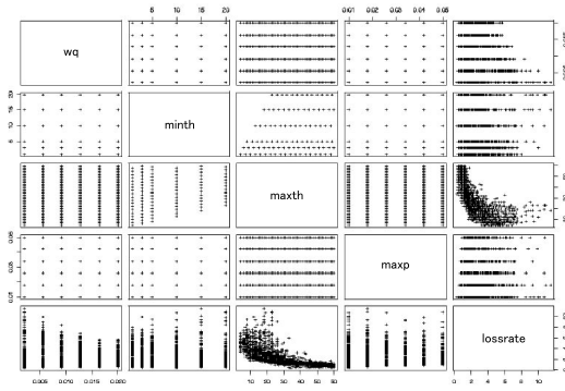
図2 REDの制御パラメータとパケット棄却率に関する多変量相関図 Fig. 2 Pair scatter plot of control parameters and packet loss probability
